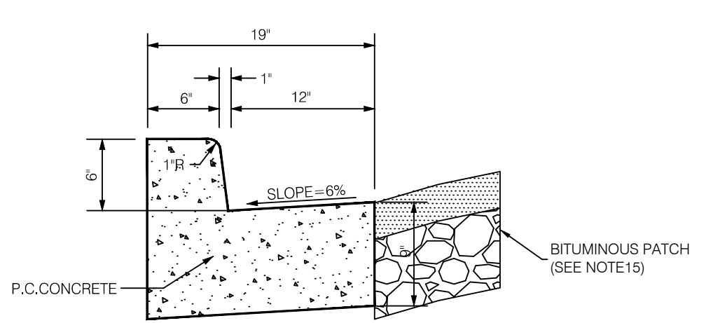
1 B-6.12 CURB AND GUTTER N.T.S.
