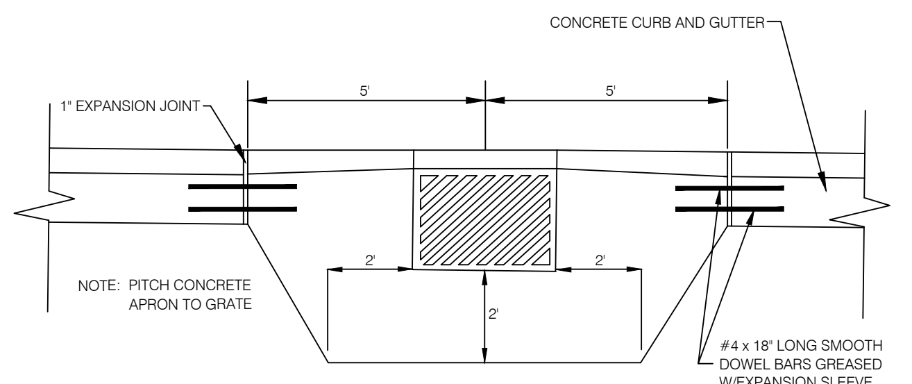
2 CURB INLET APRON DETAIL N.T.S.
